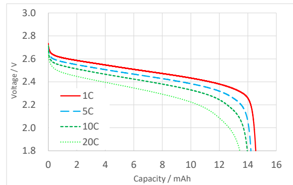
放电特性
