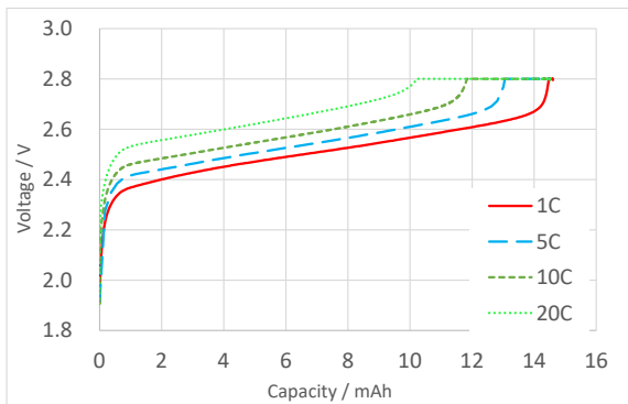
充电特性
